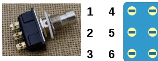
バッファードバイパス (Buffered Bypass)
