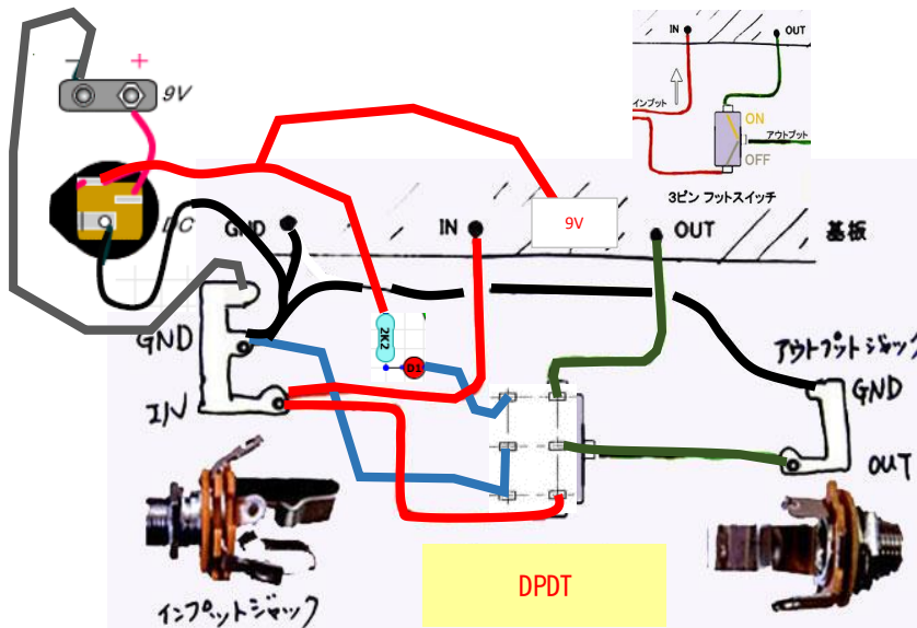
トウルーパーバイパス (TrueBypass)
