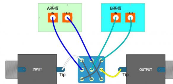
2in1ペダルでの A/B 接続順切替スイッチ実体配線図(3PDT)
